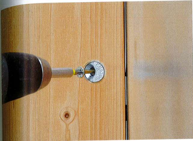
Der »T-Joint 20« von KNAPP ist ein universeller Holzverbinder, der sich vielfältig anwenden lässt.
