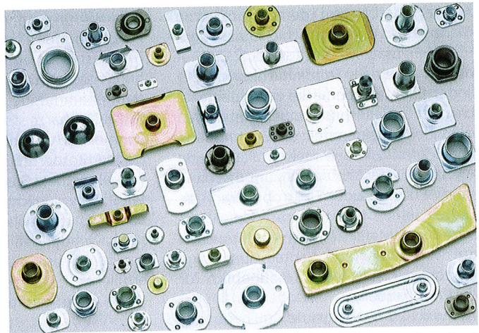
Das umfangreiche Fertigungsprogramm von LIMBACH sowie Sonderanfertigungen ermöglichen für jede Anwendung die passende Mutter.
